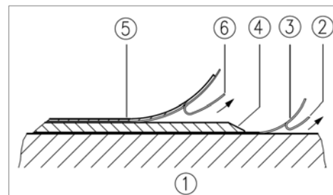
Abb. 1: Montage des Magnetbandes
