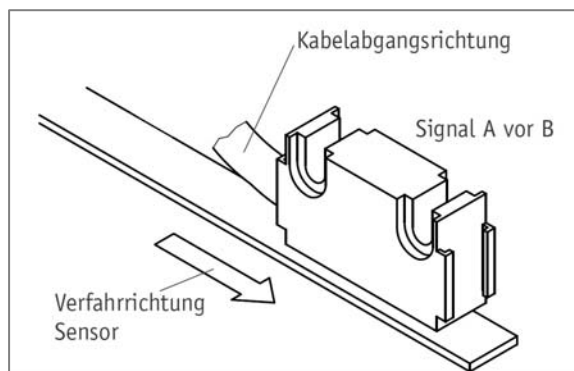
Abb. 6: Definition der Zählrichtung / Montage
