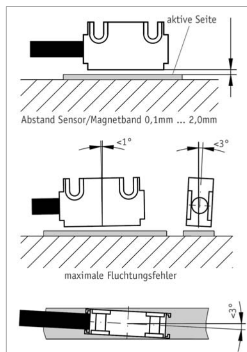
Abb. 7: Ausrichtung des Sensors
