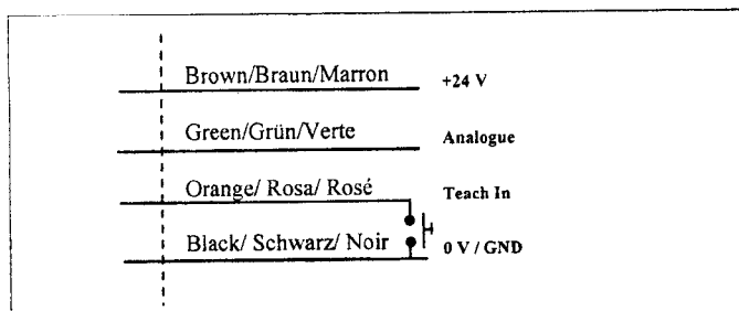
Wiring/Anschlüsse/Raccordement électrique
