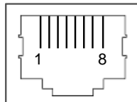
E1/T1 RJ-45 Cable Connector
