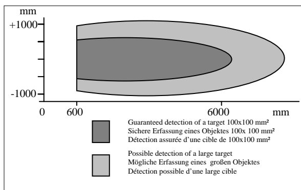
Erfassungsbereich/ Detection range/ Plage de détection mm
