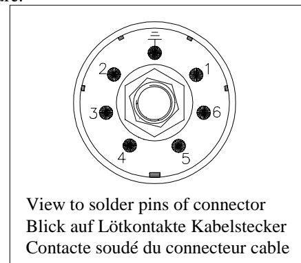
Wiring/Anschlüsse/Raccordement électrique
